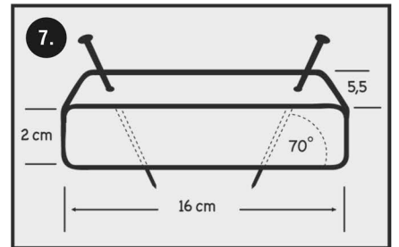
7. Skizze für DIY-Fixier-Klotz Maße Scheme for DIY-fixing-block dimensions
